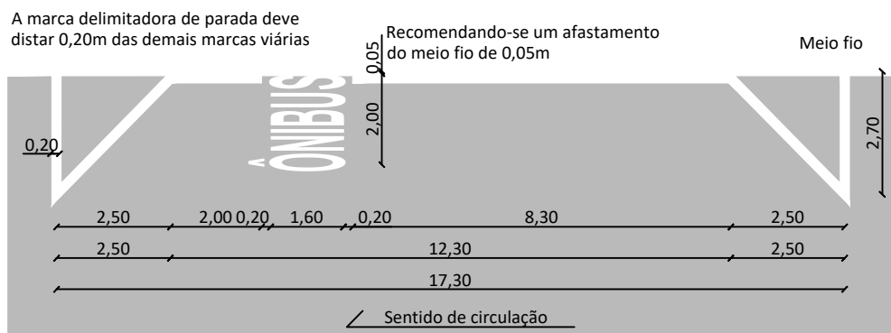
Detalhe Sinalização horizontal Esc. 1:150
