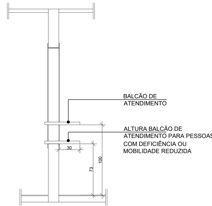
Balcão de atendimento Sem escala
