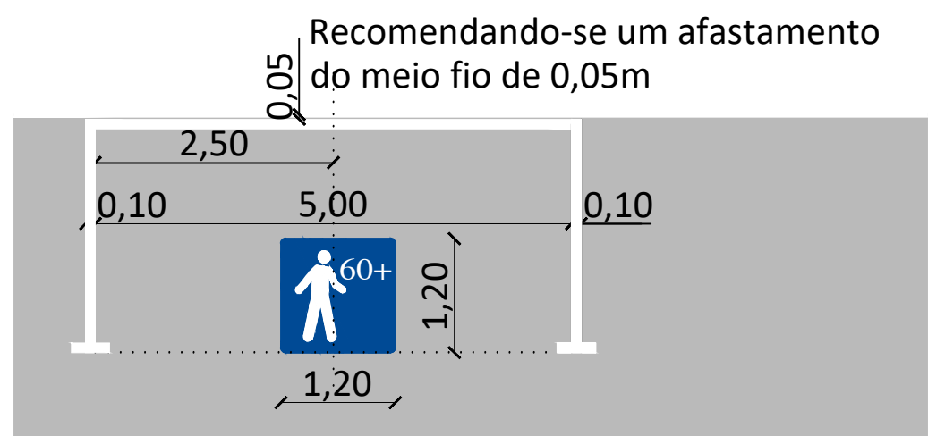
Detalhe Sinalização horizontal Sem escala
