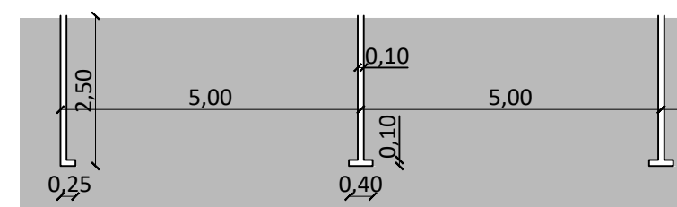
Detalhe Sinalização horizontal Esc. 1:100
