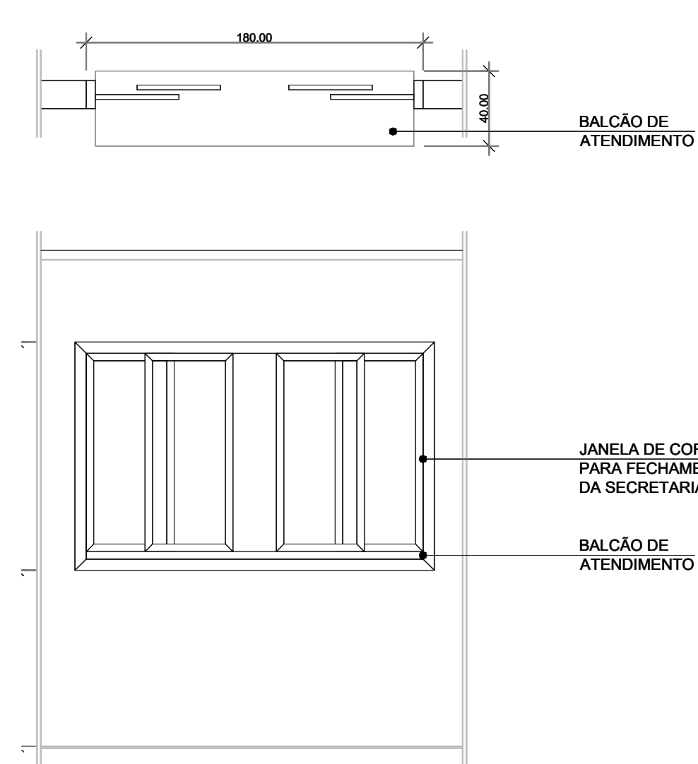
Detalhe Sinalização Vertical Esc. 1:200
