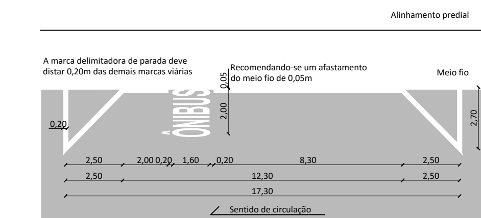
Detalhe Sinalização horizontal Esc. 1:150
