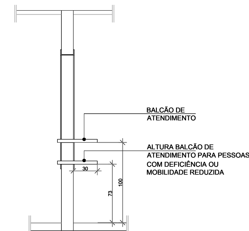
Detalhe Sinalização Vertical Esc. 1:200
