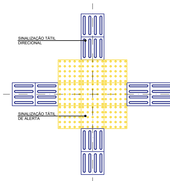
Composição da sinalização tátil de alerta e direcional Esc. 1:100
