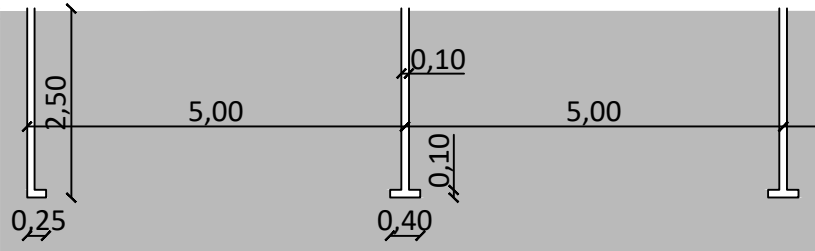
Detalhe Sinalização horizontal Esc. 1:100
