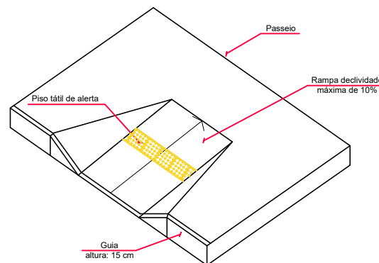
Composição da sinalização tátil de alerta e direcional da rampa Esc. 1:100
