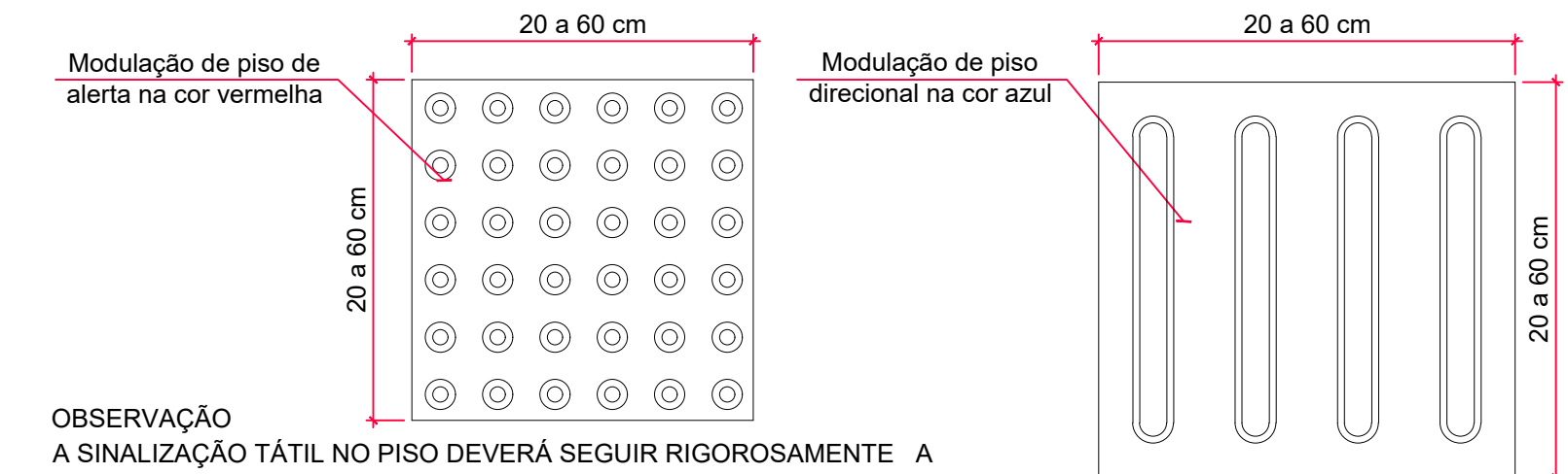
Composição da sinalização tátil de alerta e direcional Esc. 1:100
