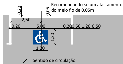
Detalhe Sinalização horizontal Esc. 1:100
