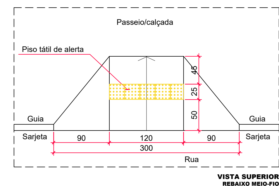
Composição da sinalização tátil de alerta e direcional da rampa Esc. 1:100
