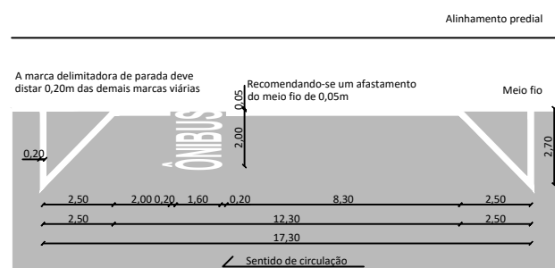
Detalhe Sinalização horizontal Esc. 1:150
