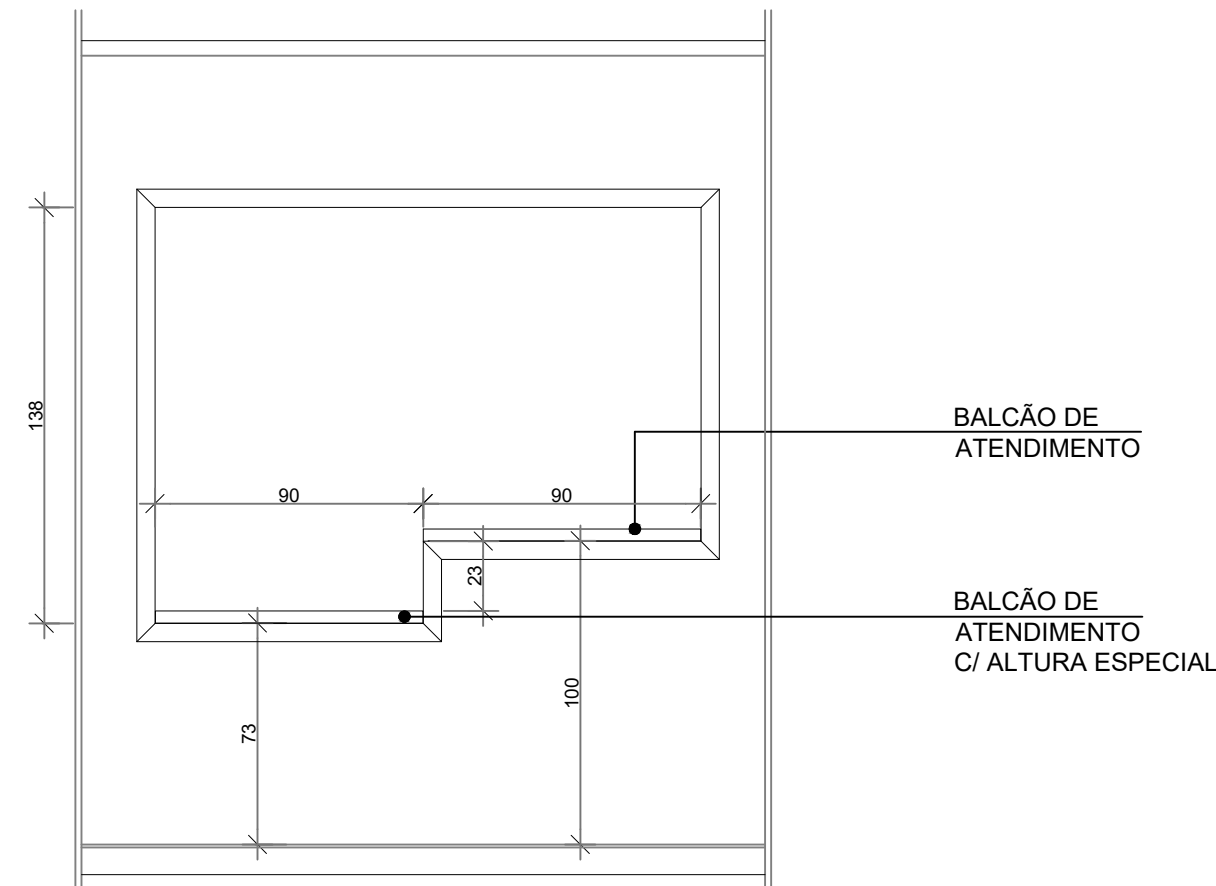
Balcão de atendimento Sem escala
