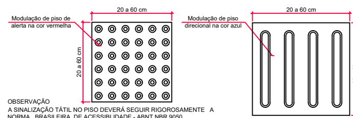
Composição da sinalização tátil de alerta e direcional Esc. 1:100
