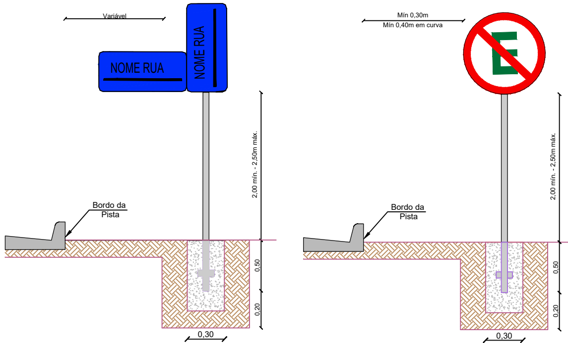
Detalhe Sinalização Vertical Sem escala
