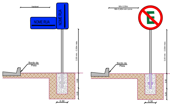
Detalhe Sinalização Vertical Sem escala
