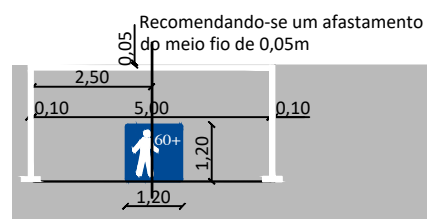
Detalhe Sinalização horizontal Esc. 1:100
