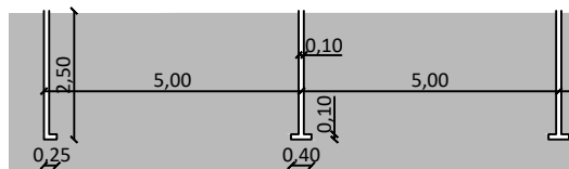
Detalhe Sinalização horizontal Esc. 1:100
