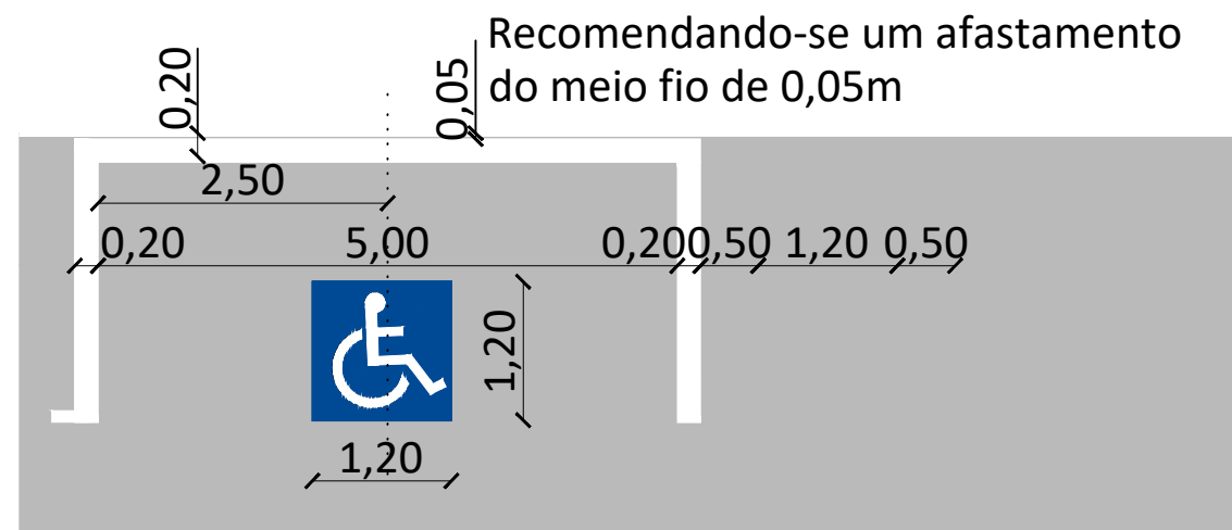
Detalhe Sinalização horizontal Sem escala
