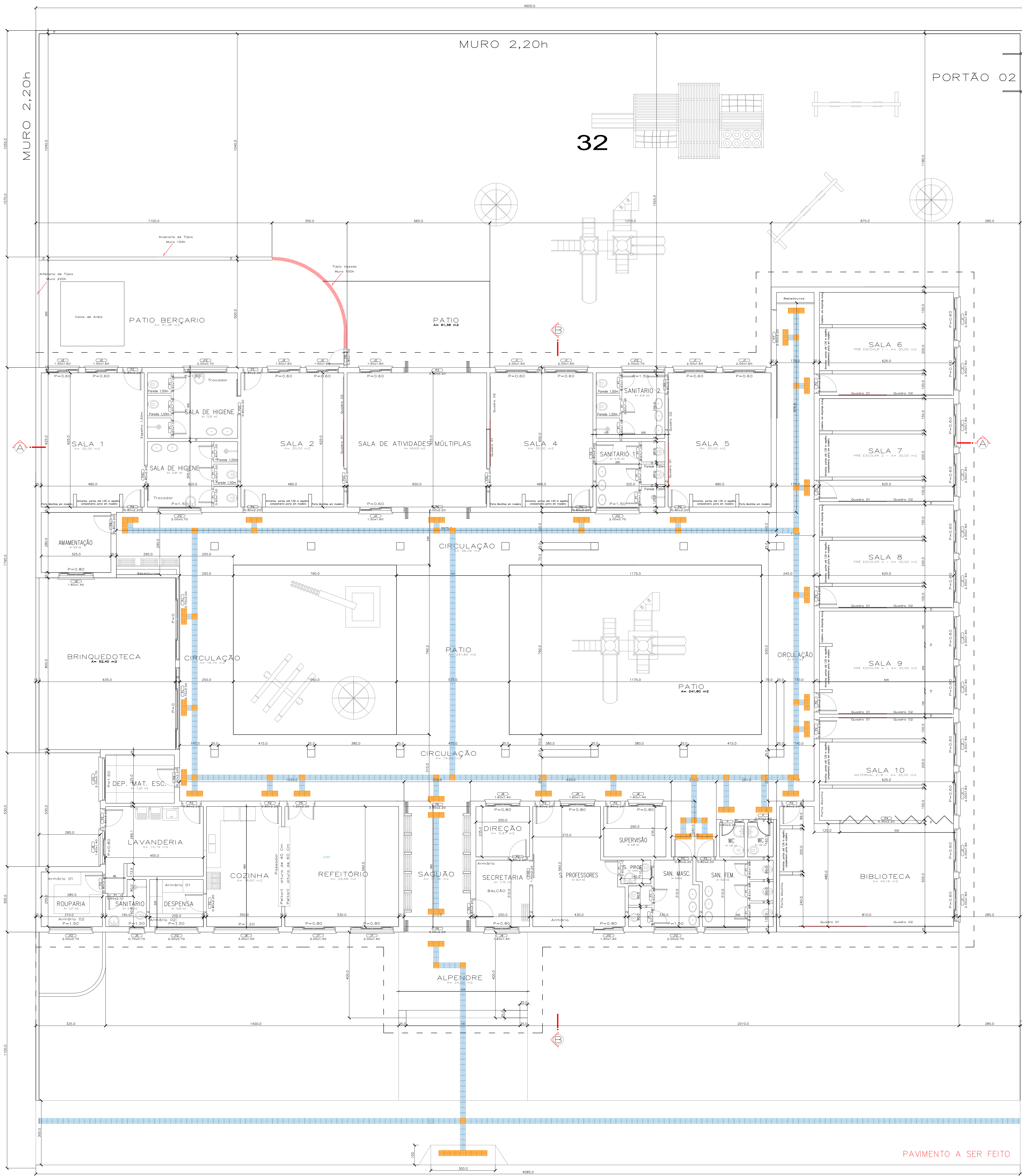
PLANTA BAIXA
