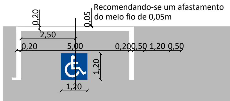
Detalhe Sinalização horizontal Esc. 1:100
