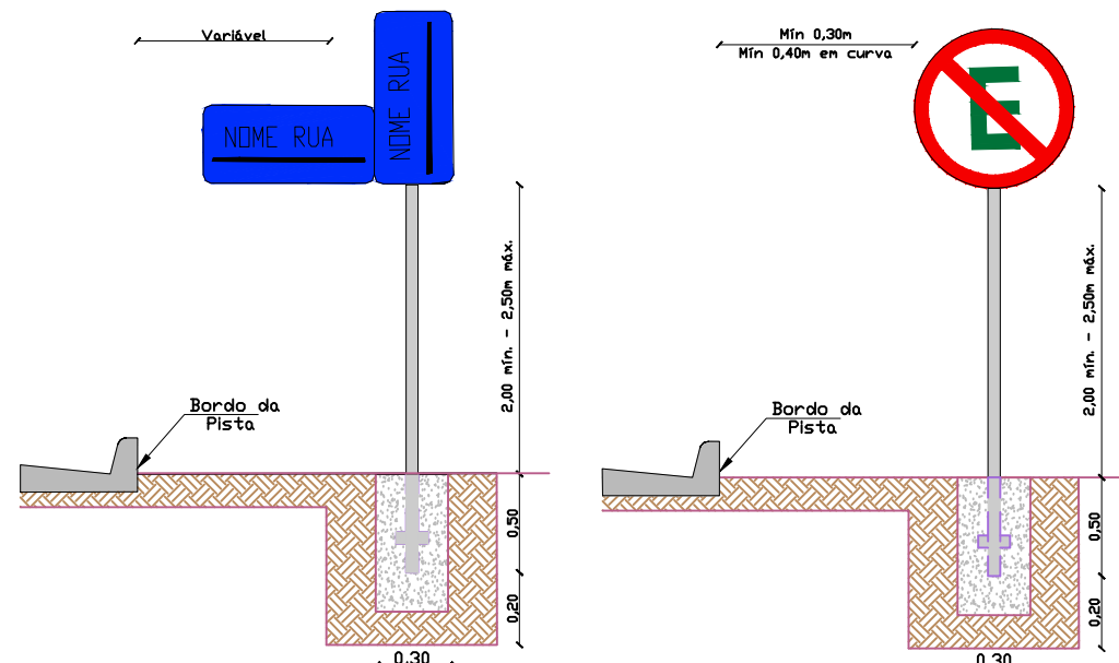
Detalhe Sinalização Vertical Sem escala
