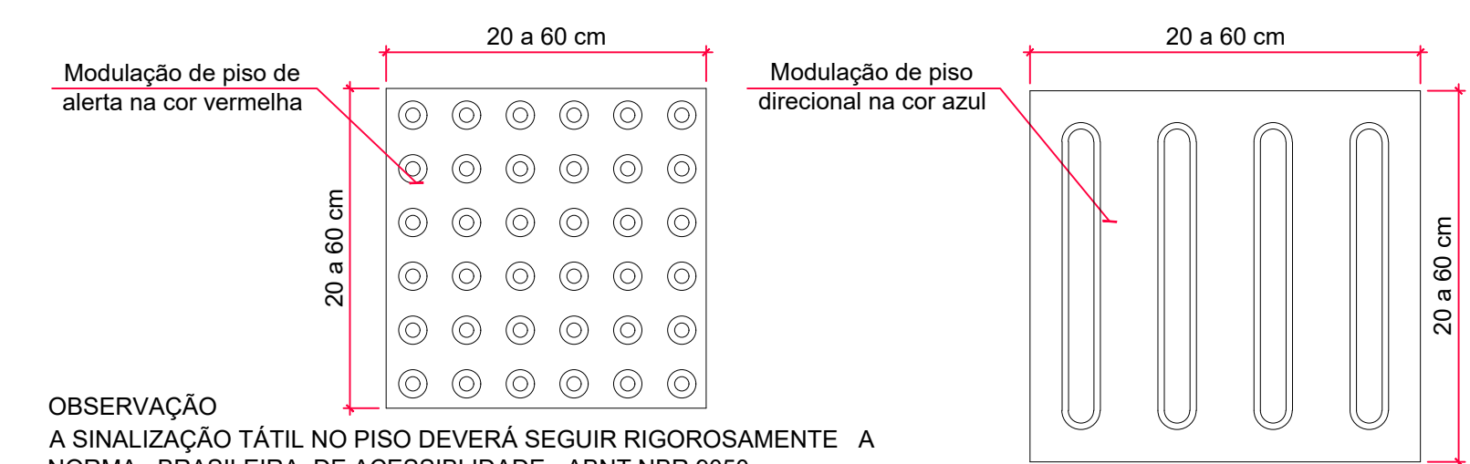
Composição da sinalização tátil de alerta e direcional Esc. 1:100
