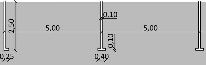
Detalhe Sinalização horizontal Esc. 1:100
