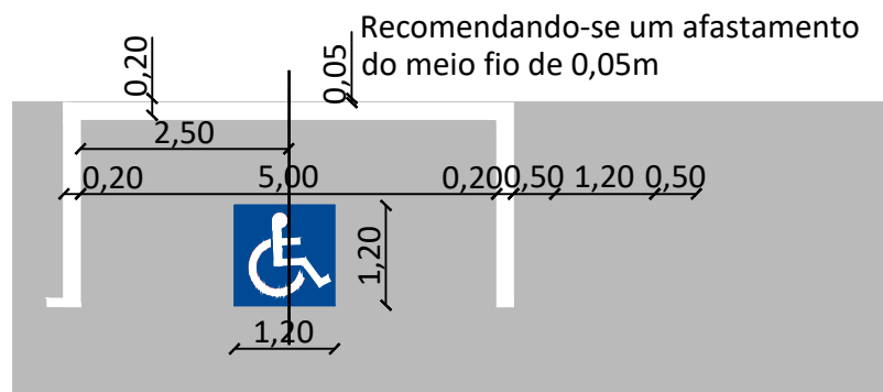
Detalhe Sinalização horizontal Esc. 1:100
