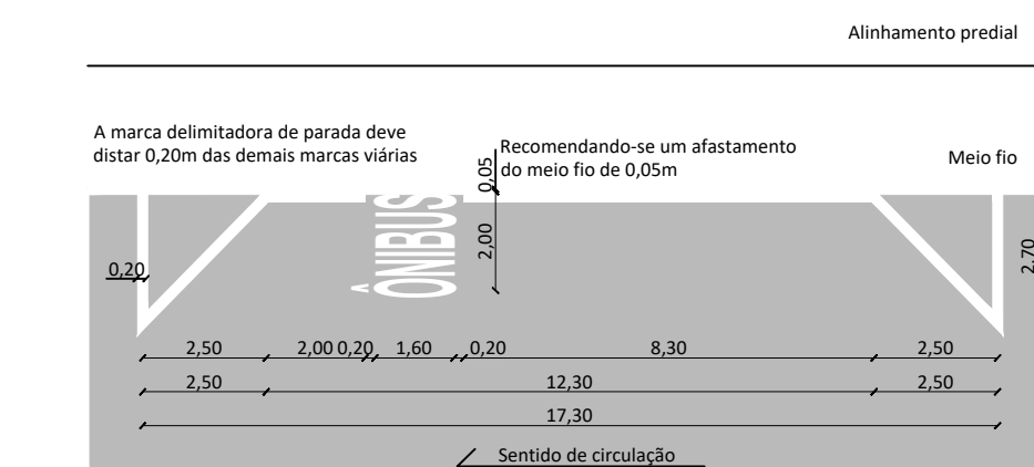
Detalhe Sinalização horizontal Esc. 1:150
