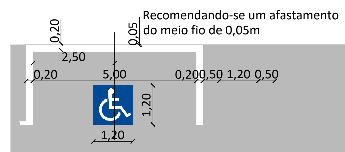
Detalhe Sinalização horizontal Sem escala
