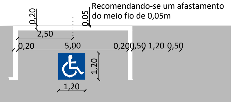
Detalhe Sinalização horizontal Esc. 1:100
