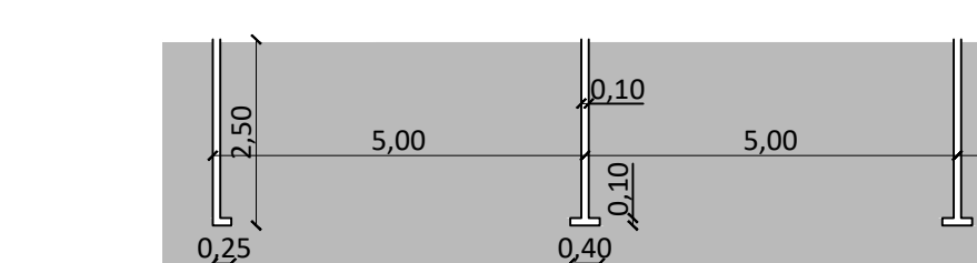
Detalhe Sinalização horizontal Esc. 1:100
