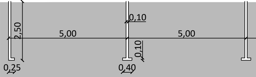
Detalhe Sinalização horizontal Esc. 1:100
