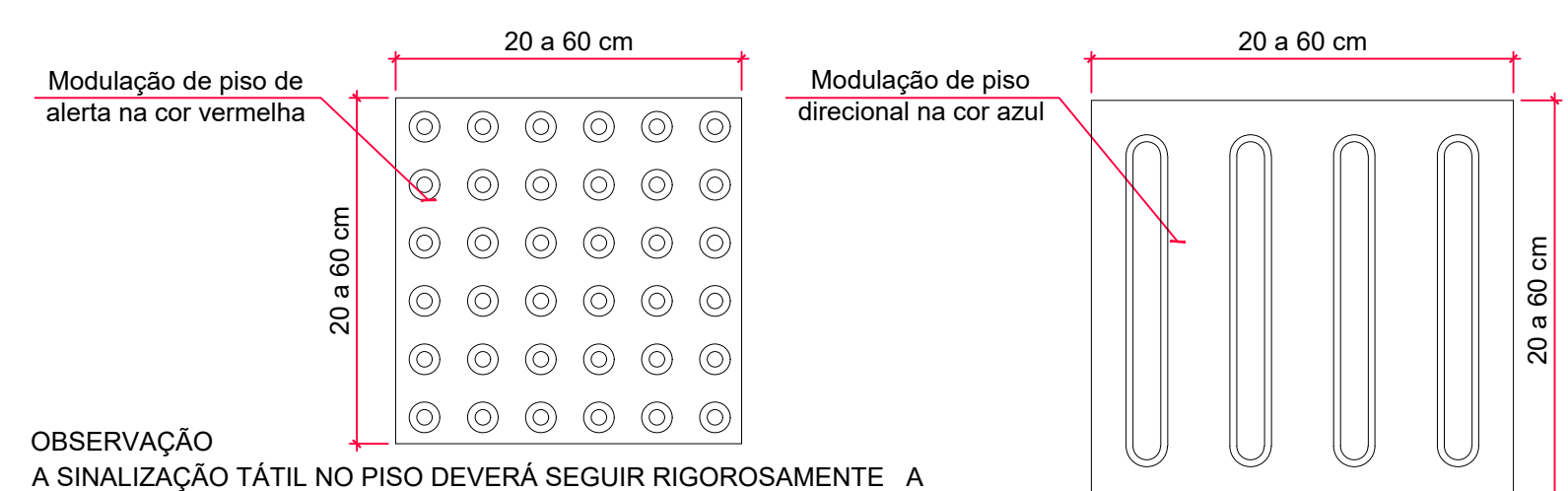
Detalhe Sinalização horizontal Esc. 1:150
