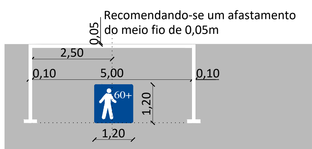
Detalhe Sinalização horizontal Sem escala
