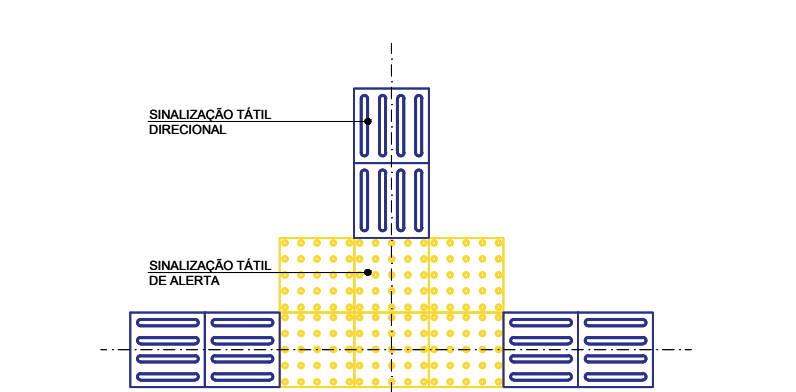
Detalhe Sinalização tátil e visual Esc. 1:100
