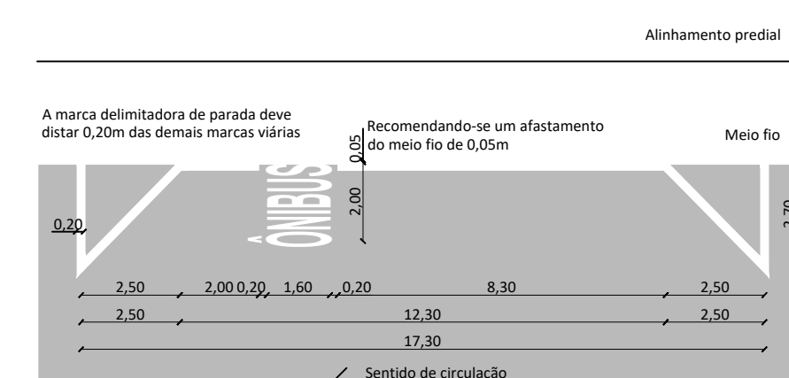
Detalhe Sinalização horizontal Esc. 1:150
