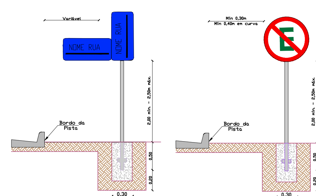
Detalhe Sinalização Vertical Sem escala
