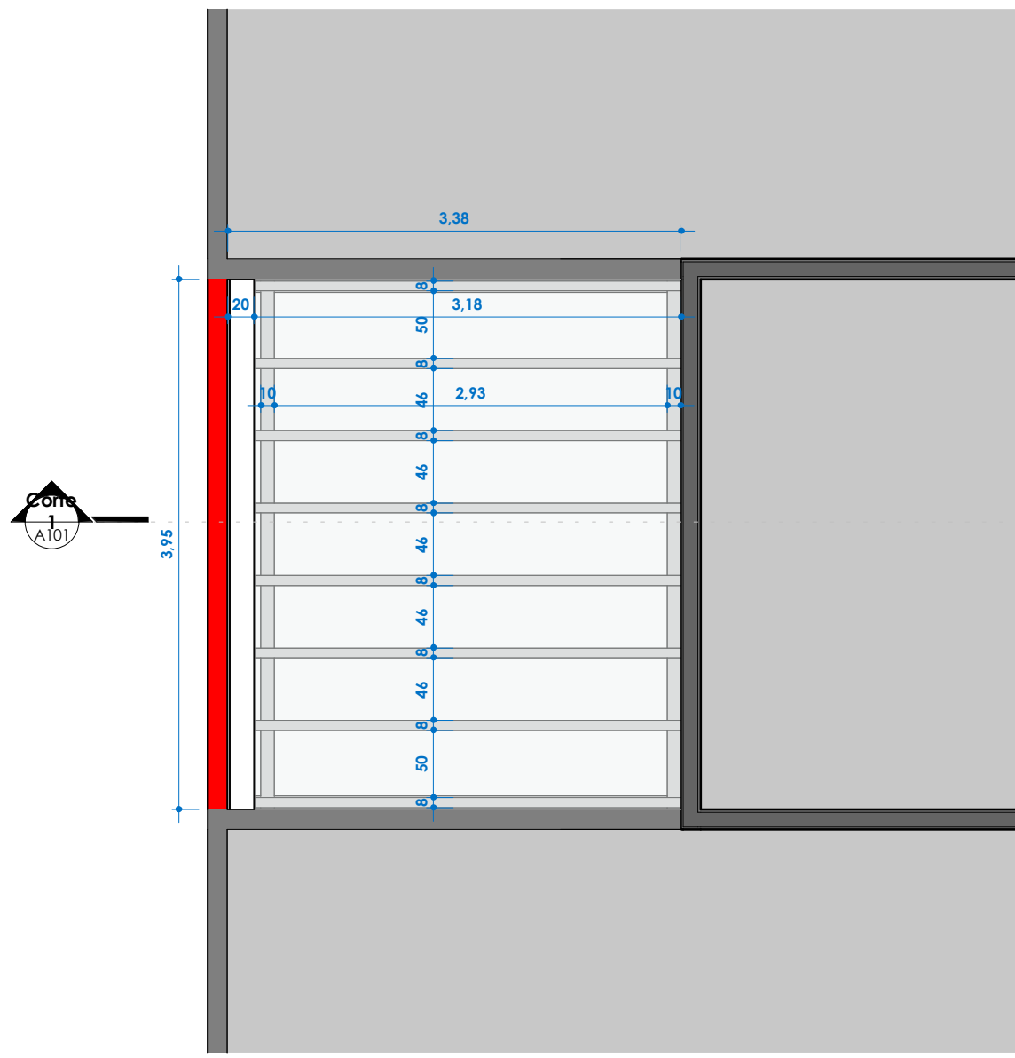
1 Superior 1 : 50
