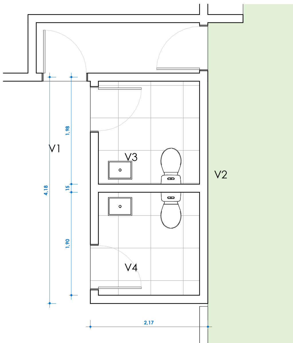
2 FORMA 1 : 40
