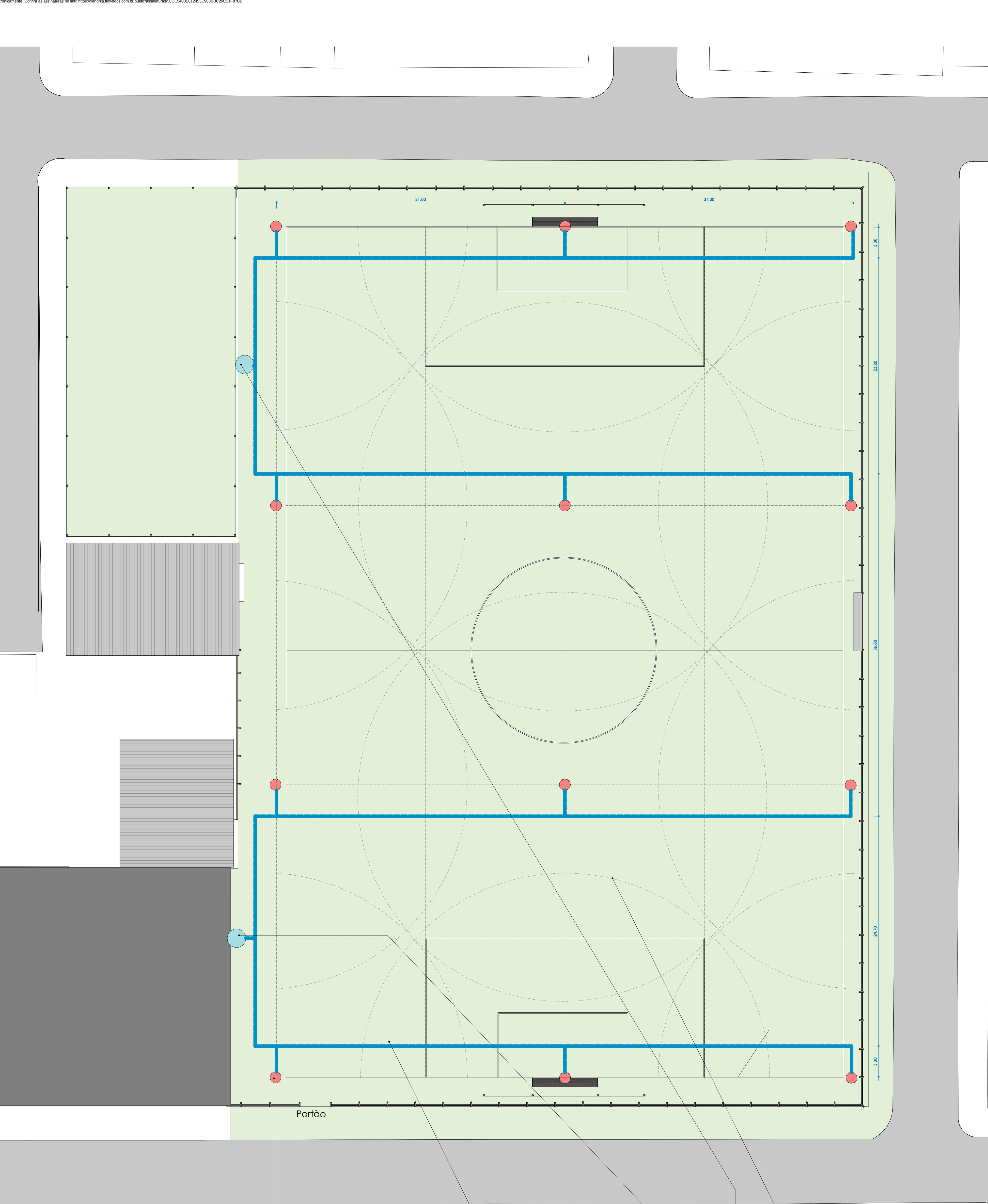
Irrigação ESC: 1 : 200 Aspersor Rain Bird® 8005 Tubulação Água Poço Artesiano Alcance do aspersor água
