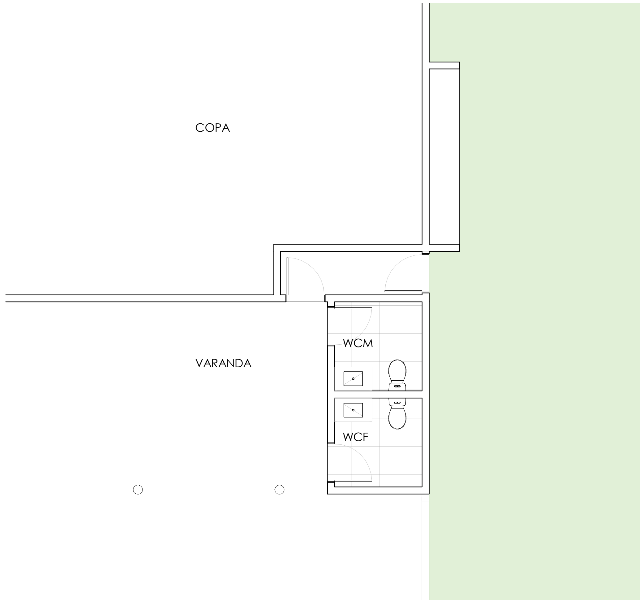
1 Planta Baixa Banheiros 1 : 50
