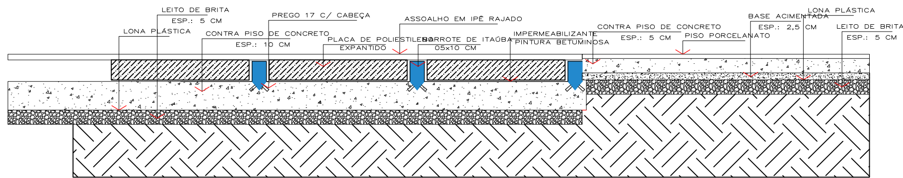
DETALHAMENTO PISO
