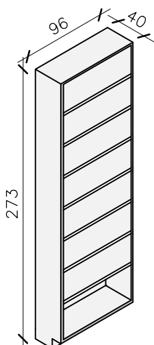
PERSPECTIVA ESCALA.....S/E
