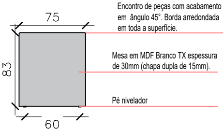
VISTA 02 ESCALA.....1/30
