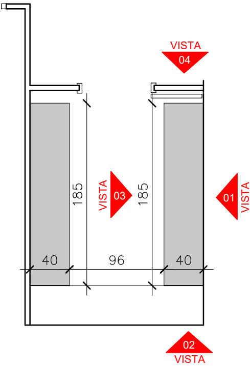
VISTA SUPERIOR
