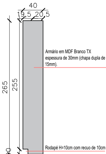
VISTA 02 ESCALA.....1/30
