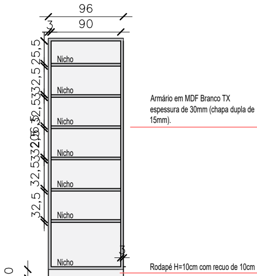
VISTA 03 ESCALA.....1/30
