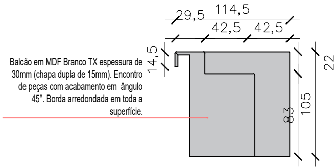
VISTA 02 ESCALA.....1/30
