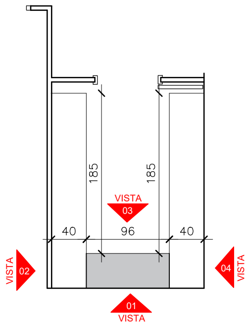
VISTA SUPERIOR ESCALA.....1/30
