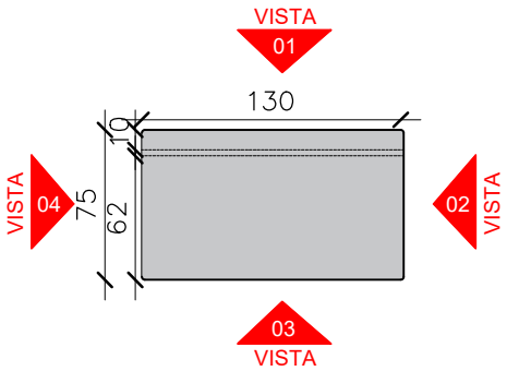
VISTA SUPERIOR ESCALA.....1/30
