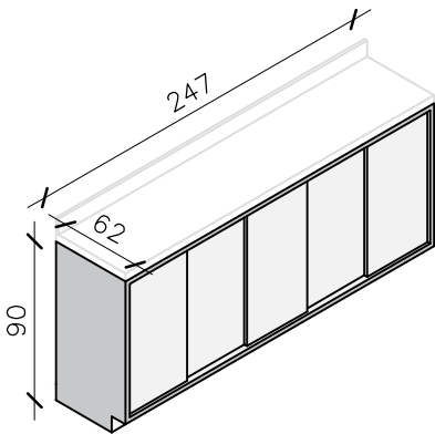
PERSPECTIVA ESCALA..... S/E
