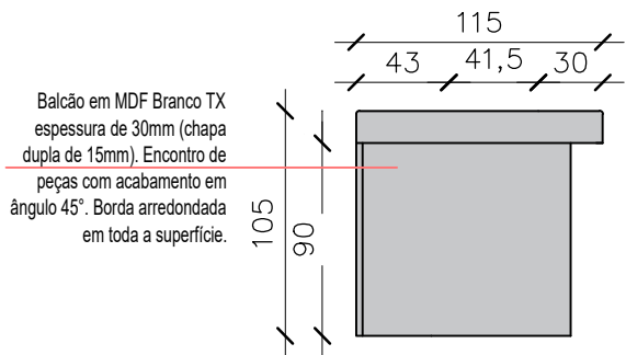
VISTA 04 ESCALA.....1/30
