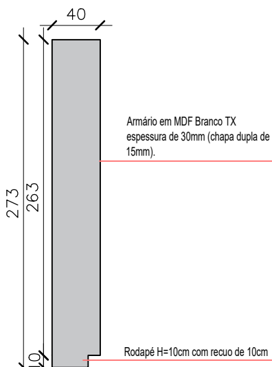
VISTA 04 ESCALA.....1/30
