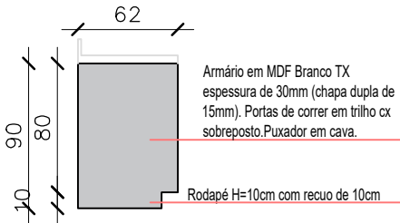
VISTA 04 ESCALA..... 1/30
