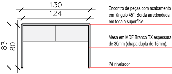
VISTA 01 ESCALA.....1/30
