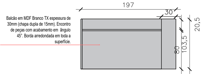
VISTA 03 ESCALA.....1/30
