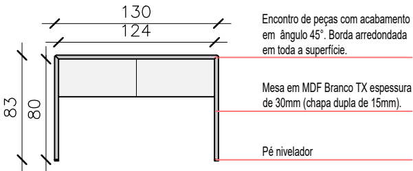
VISTA 03 ESCALA.....1/30
