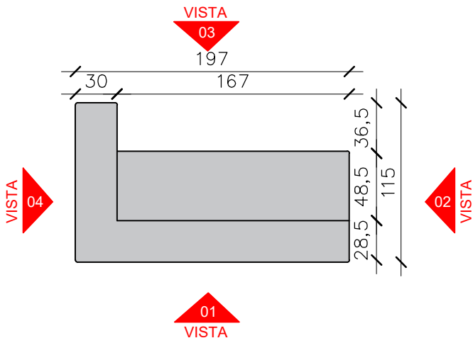
PLANTA BAIXA ESCALA.....1/30
