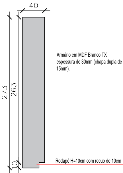
VISTA 04
