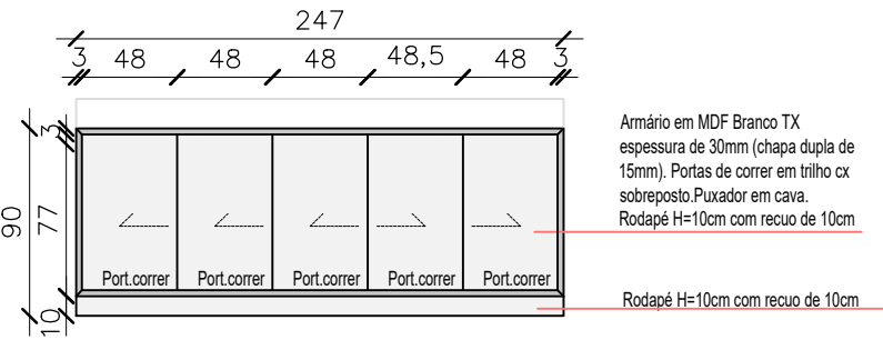
VISTA 03 ESCALA..... 1/30
