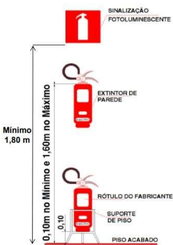
Figura 2: Detalhe da fixação do extintor de incêndio – desenho retirado da RT 14/2016.
