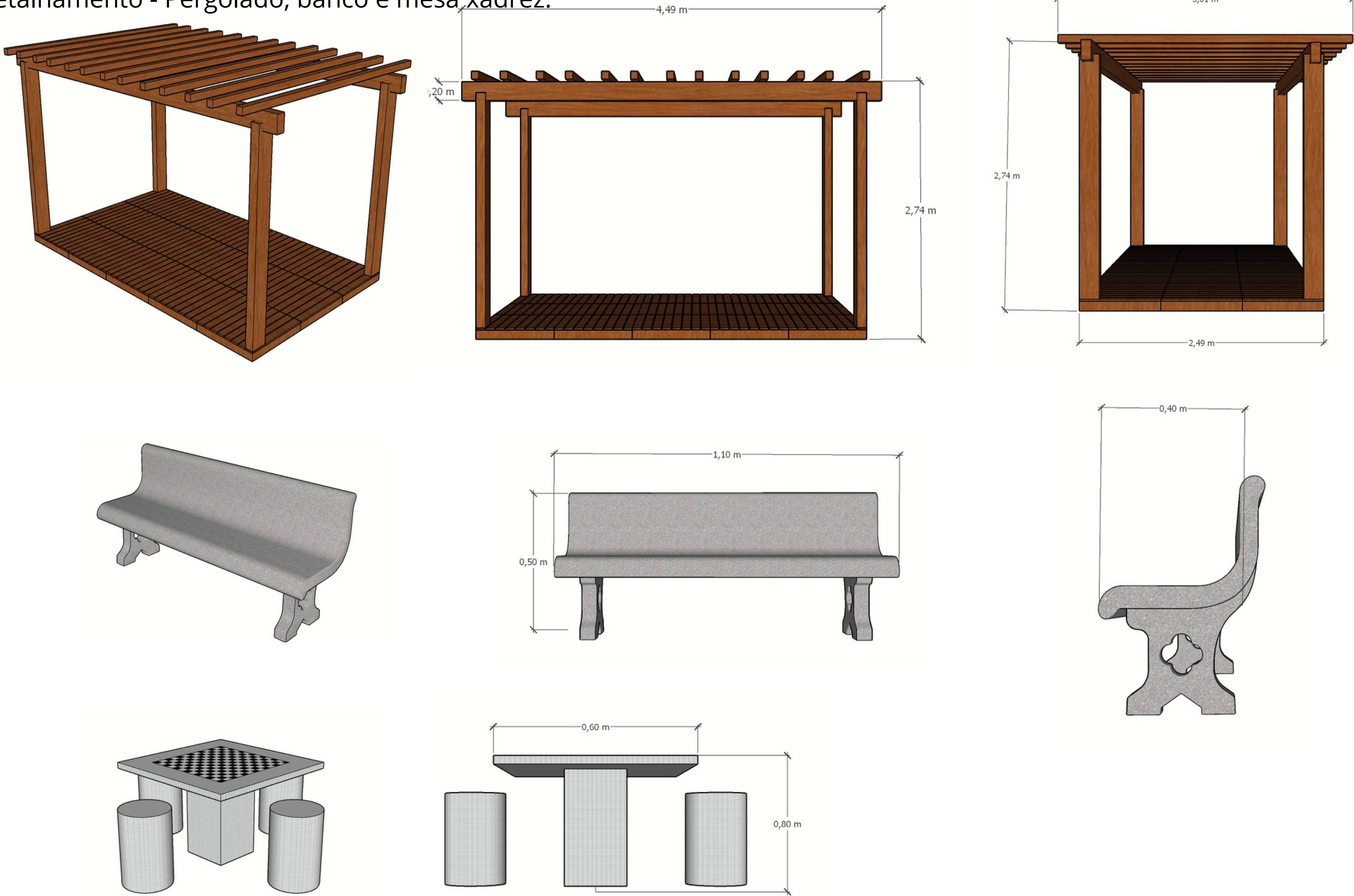
Detalhamento - Pergolado, banco e mesa xadrez.
