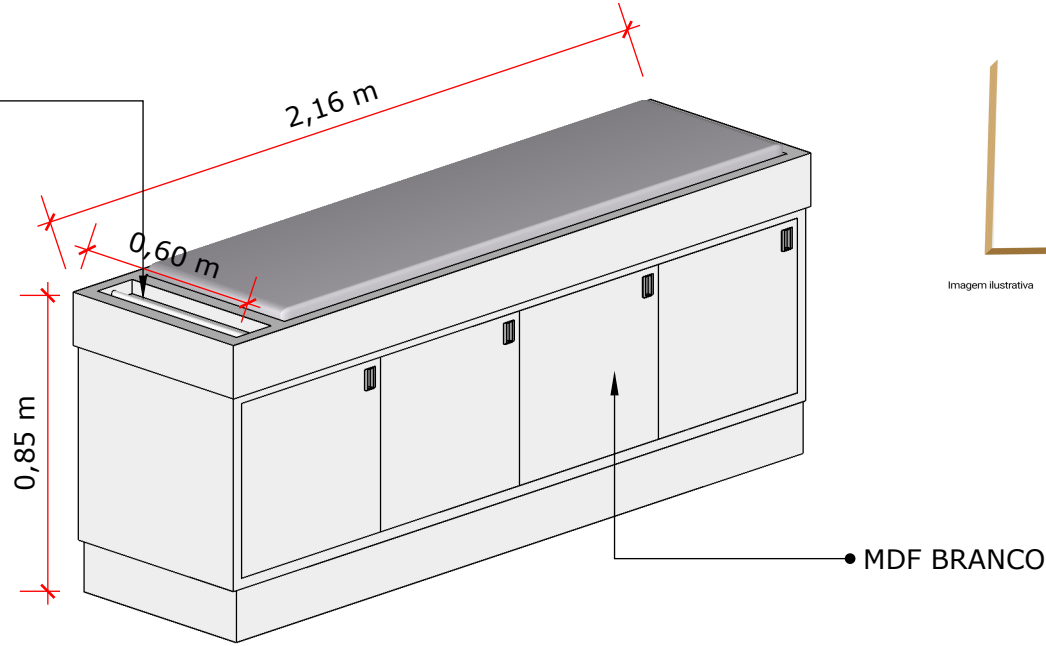
SUPORTE ROLO DE PAPEL
