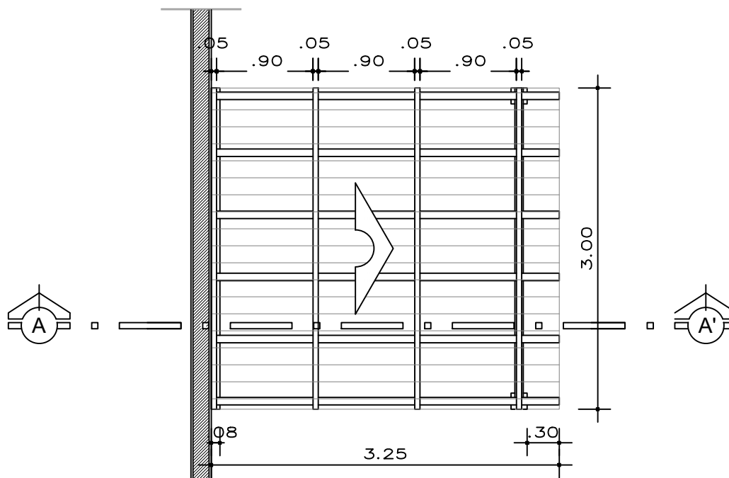
TIPO 1 - PAREDE VISTA SUPERIOR
