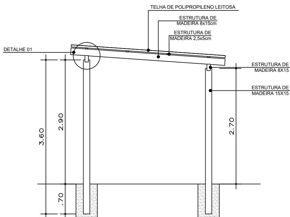
TIPO 6 - RETO solto
