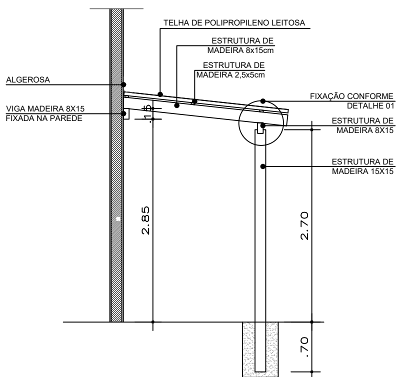
TIPO 5 - PAREDE CIRCULAÇÃO CORTE AA'
