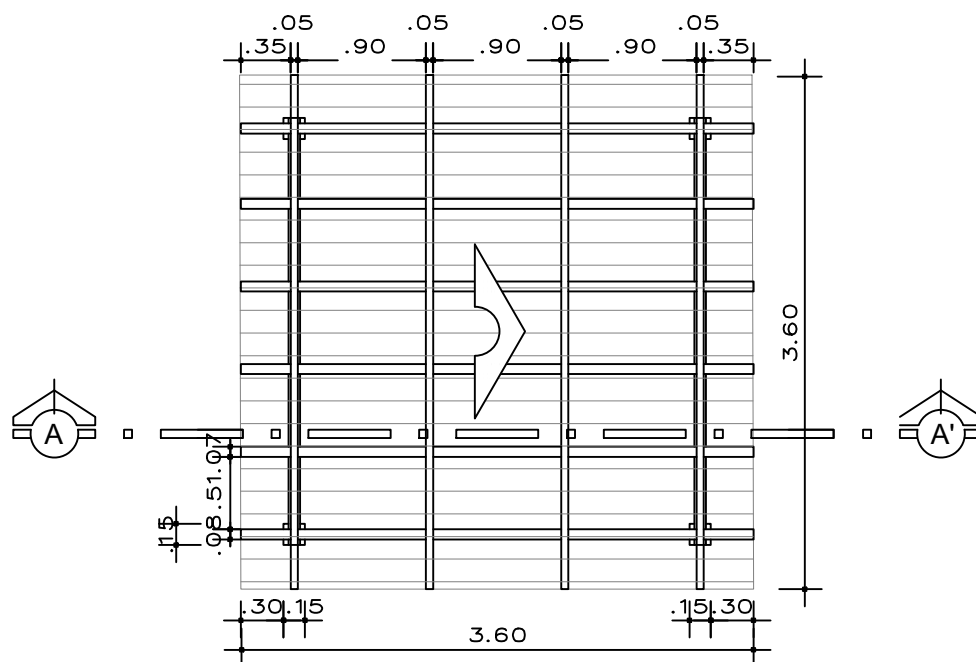
TIPO 6 - RETO solto
