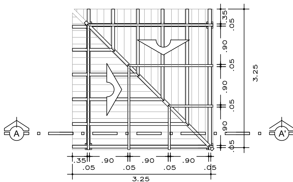
TIPO 2 - CANTO VISTA SUPERIOR
