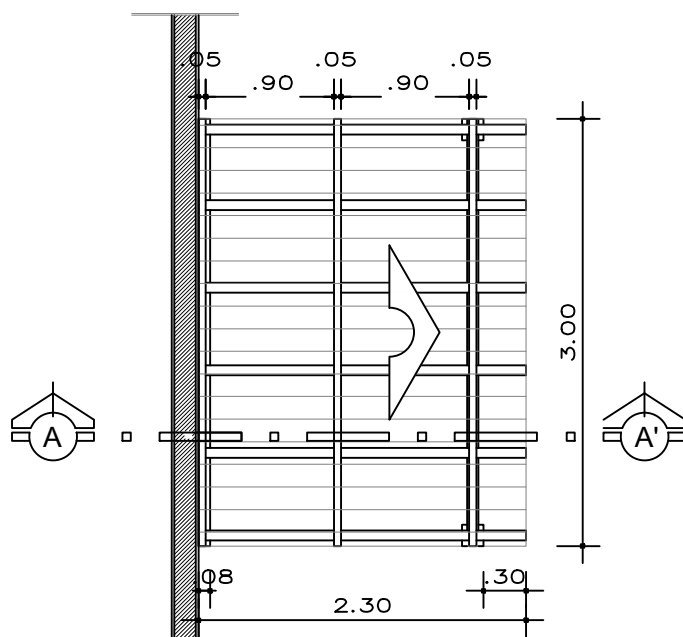
TIPO 5 - PAREDE CIRCULAÇÃO VISTA SUPERIOR
