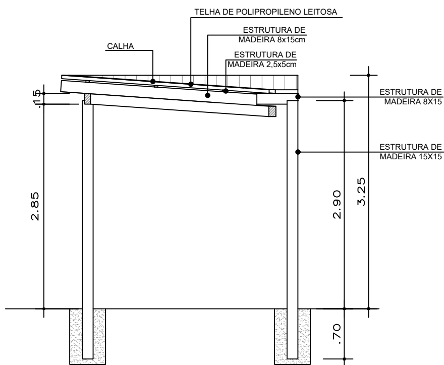
TIPO 2 - CANTO CORTE AA'
